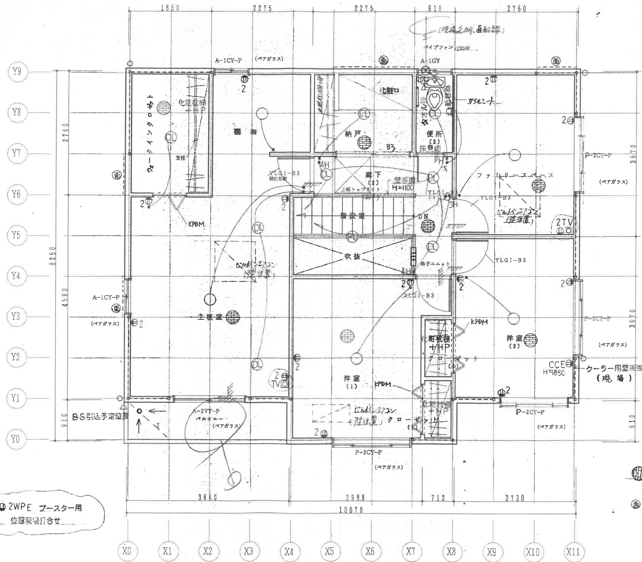
2階平面図
